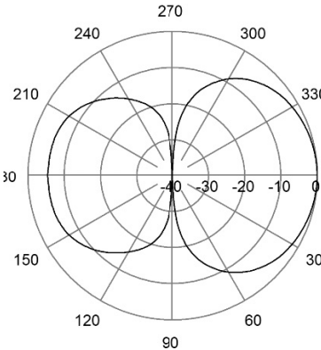
E-Plane | 225 MHz
