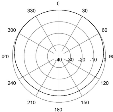
H-Plane | 225 MHz
