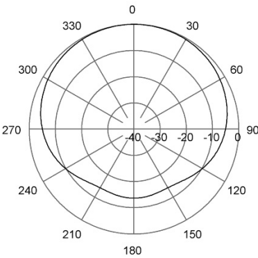
H-Plane | 153 MHz
