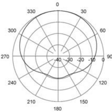
H-Plane | 61 MHz
