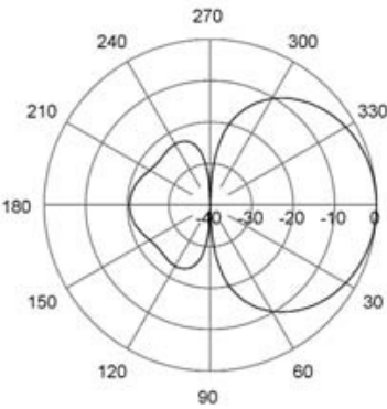
E-Plane | 61 MHz
