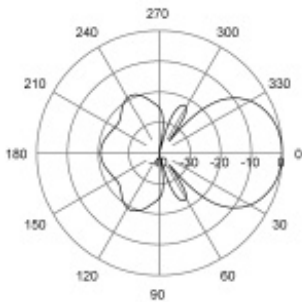
E-Plane | 767 MHz
