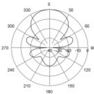
H-Plane | 767 MHz
