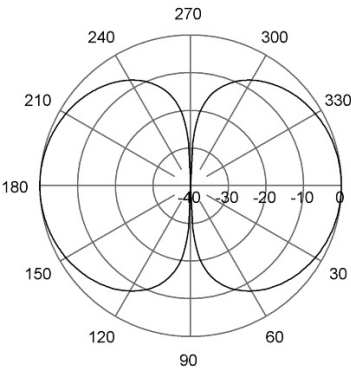
E-Plane | 165 MHz
