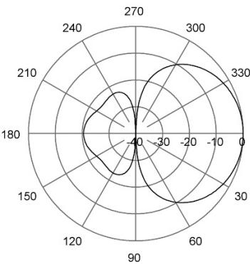
E-Plane | 71 MHz
