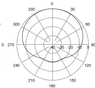
H-Plane | 71 MHz
