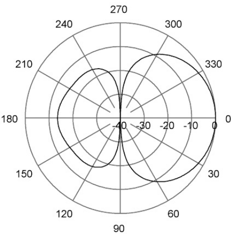
E-Plane | 400 MHz
