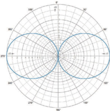
E-Plane | 155 MHz
