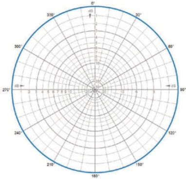
H-Plane | 155 MHz
