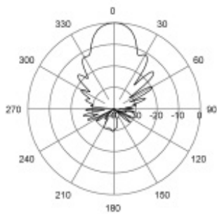
H-Plane | 1478 MHz
