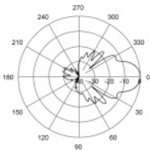
E-Plane | 1478 MHz
