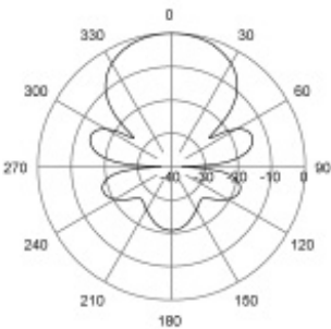
H-Plane | 875 MHz
