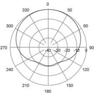
H-Plane | 72 MHz
