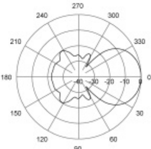
E-Plane | 436 MHz
