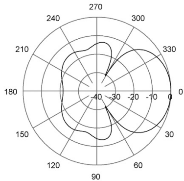
H-Plane | 390 MHz
