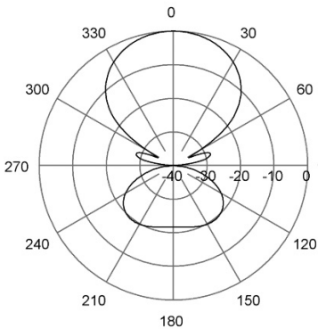
E-Plane | 390 MHz
