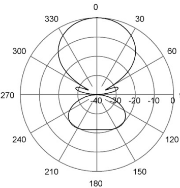
E-Plane | 180 MHz
