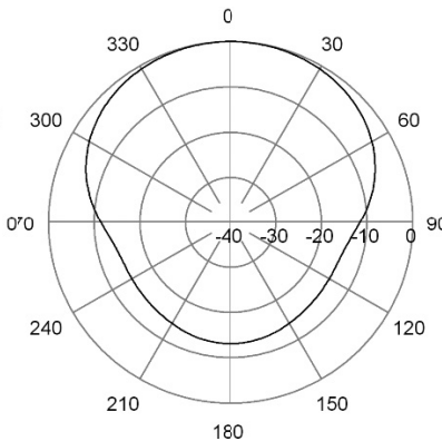
H-Plane | 96 MHz
