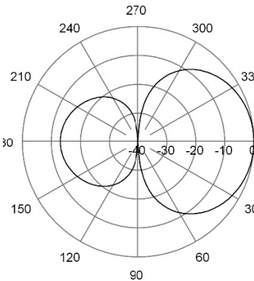
E-Plane | 96 MHz
