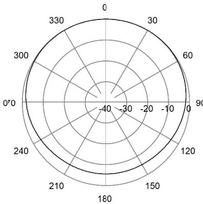
H-Plane | 405 MHz
