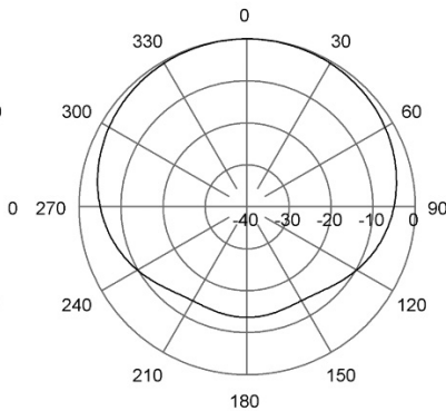
H-Plane | 49 MHz
