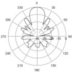
H-Plane | 435 MHz
