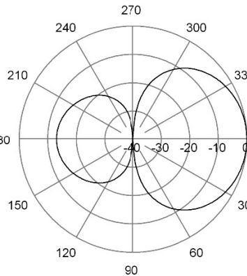
E-Plane | 155 MHz
