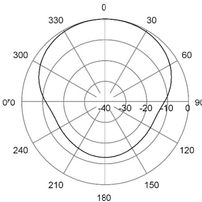
H-Plane | 155 MHz
