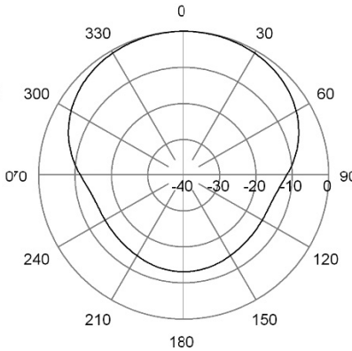
H-Plane | 128 MHz
