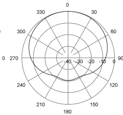
H-Plane | 82 MHz
