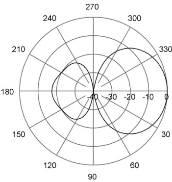
E-Plane | 160 MHz
