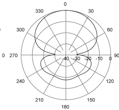
H-Plane | 160 MHz
