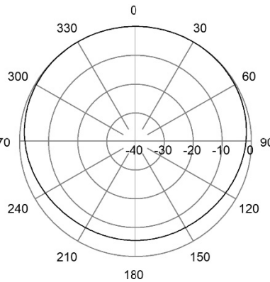
H-Plane | 148 MHz
