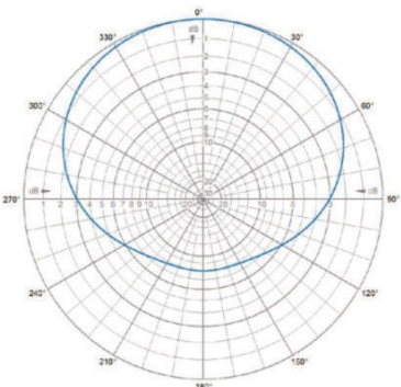
H-Plane | 405 MHz
