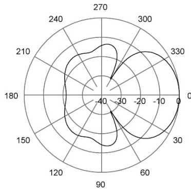
H-Plane | 440 MHz
