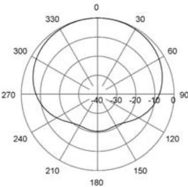
H-Plane | 160 MHz
