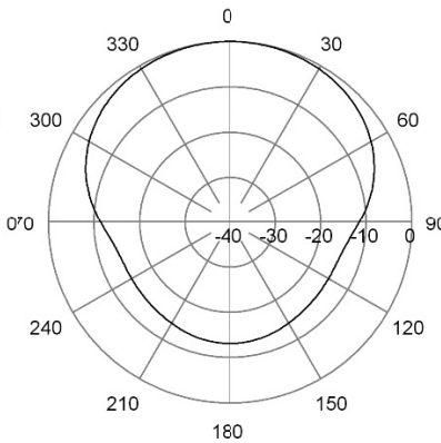
H-Plane | 73 MHz
