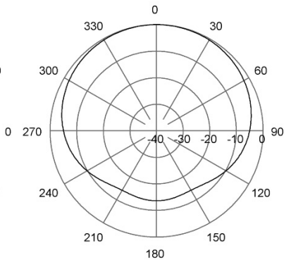
H-Plane | 102 MHz
