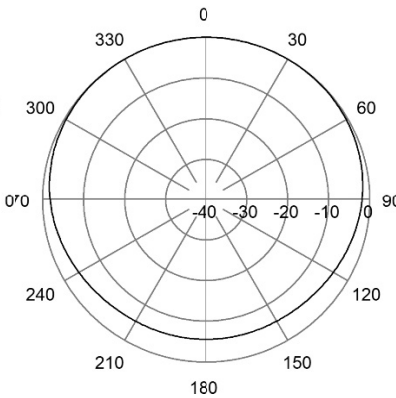
H-Plane | 68 MHz
