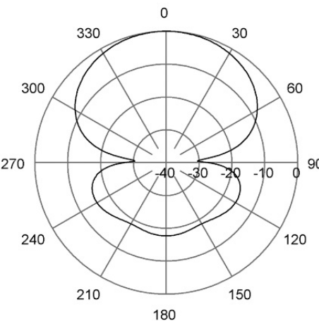
H-Plane | 445 MHz
