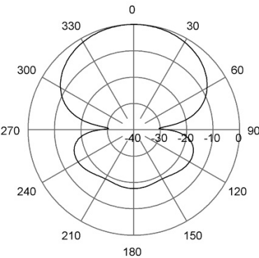
H-Plane | 390 MHz
