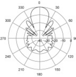
H-Plane | 580 MHz
