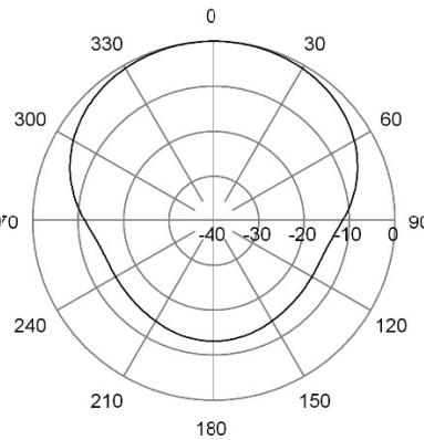
H-Plane | 120 MHz
