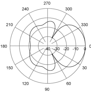
H-Plane | 110 MHz
