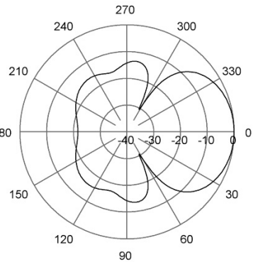
H-Plane | 455 MHz
