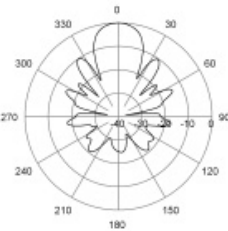
H-Plane | 455 MHz
