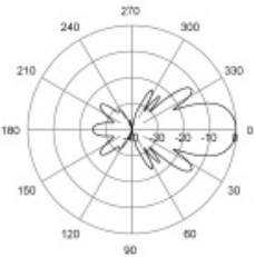
E-Plane | 455 MHz
