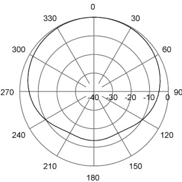
H-Plane | 72 MHz
