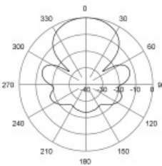
H-Plane | 220 MHz
