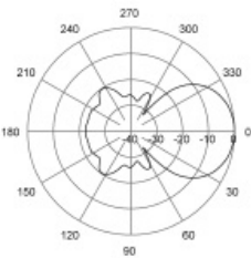
E-Plane | 220 MHz
