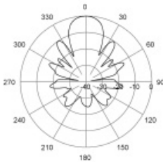
H-Plane | 770 MHz
