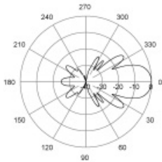
E-Plane | 770 MHz
