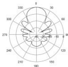
H-Plane | 445 MHz
