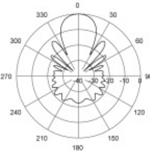
H-Plane | 860 MHz
