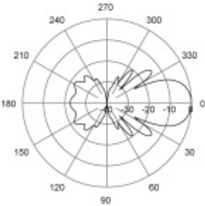
E-Plane | 860 MHz
