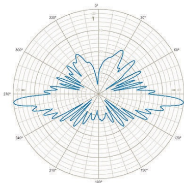
E-Plane | 875 MHz | 6°
