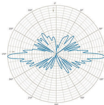
E-Plane | 875 MHz | 3°
