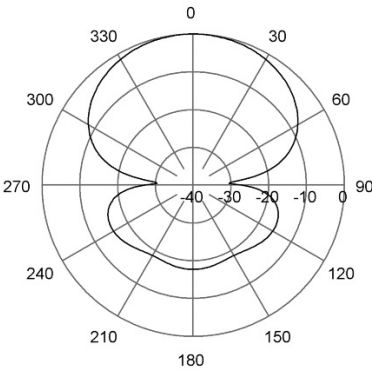
H-Plane | 2400 MHz
