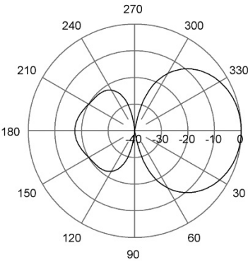
E-Plane | 2400 MHz
