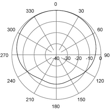
H-Plane | 82 MHz
