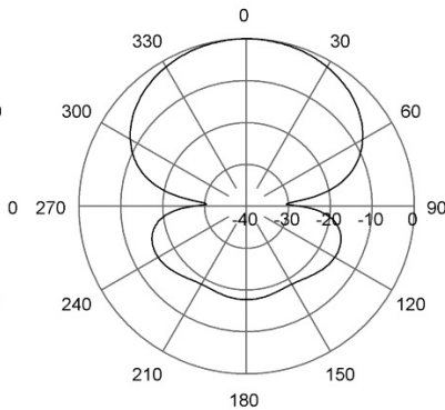
H-Plane | 330 MHz
