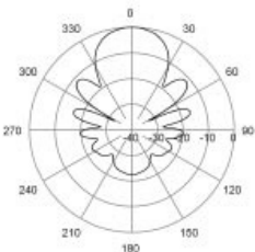
H-Plane | 395 MHz
