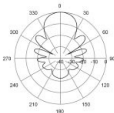
H-Plane | 418 MHz
