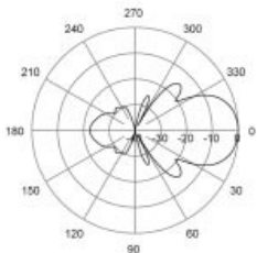
E-Plane | 418 MHz
