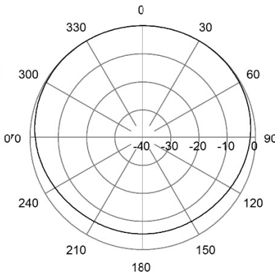
H-Plane | 193 MHz
