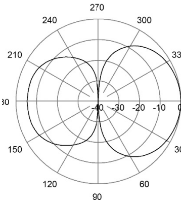
E-Plane | 193 MHz
