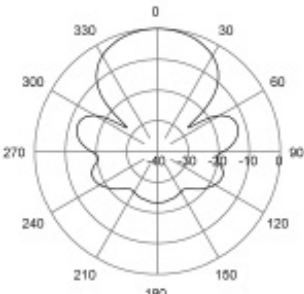
H-Plane | 330 MHz
