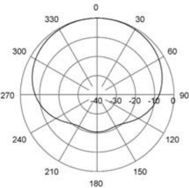
H-Plane | 49 MHz
